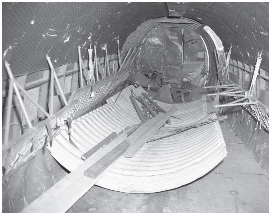
L'avion CF-DXR accidenté de la Hollinger Ungava Transport, 18 octobre 1951. Archives nationales à Sept-Îles, fonds Compagnie minière IOC (P21,717 et P21,723). Photographie non identifiée.
